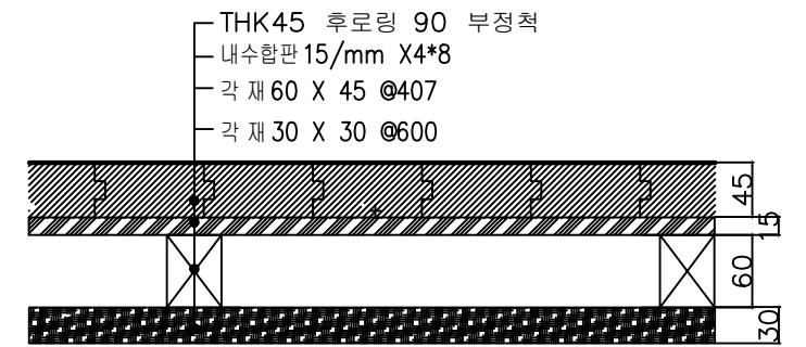
바닥 마루 단면 상세
