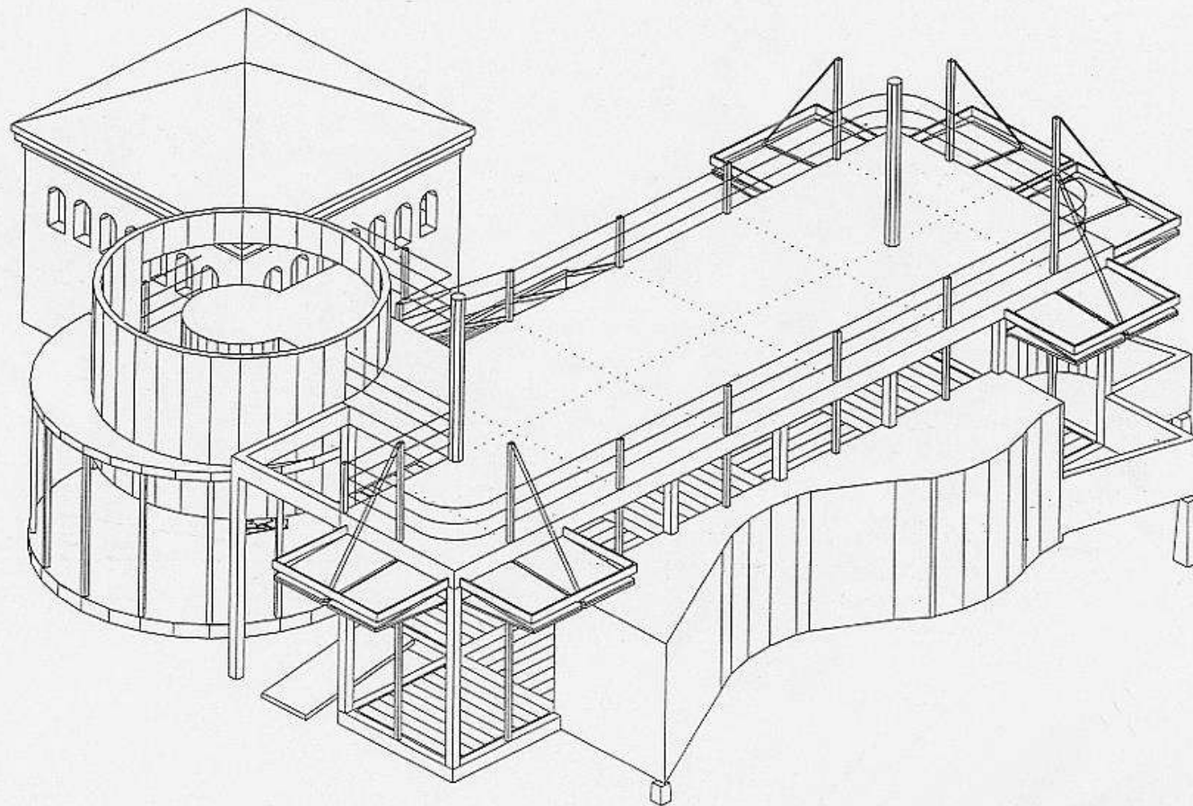
PADIGLIONE DELLA REPUBBLICA DI COREA AI GIARDINI DELLA BIENNALE. VENEZIA, APRILE 1994 VISTA ASSONOMETRICA
