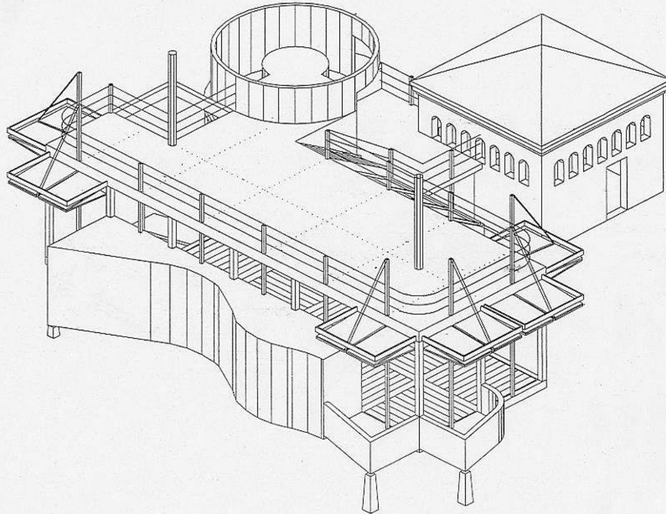
PADIGLIONE DELLA REPUBBLICA DI COREA AI GIARDINI DELLA BIENNALE. VENEZIA, APRILE 1994 VISTA ASSONOMETRICA
